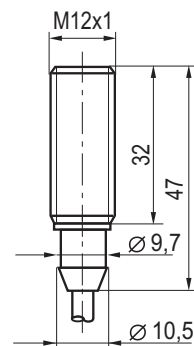
Габаритный чертеж
